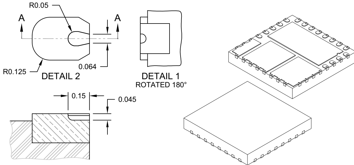
SECTION A-A
