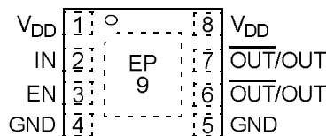
MCP14A0901/MCP14A0902 2 x 3 TDFN*
