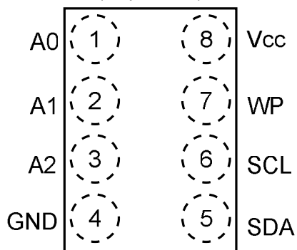
8-ball VFBGA
